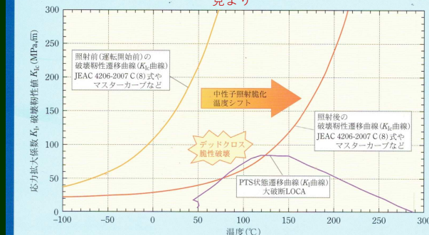
加圧熱衝撃 (PTS) 評価 (破壊靱性遷移曲線と PTS 状態遷移曲線)
