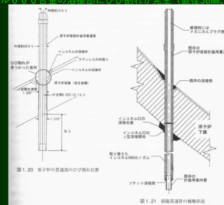
図 1.21 損傷貫通管の補修状況
