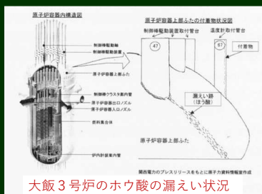
大飯3号炉のホウ酸の漏えい状況
