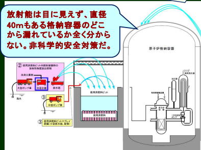
対策イメージ(大容量泡放水砲システムによる放水)
